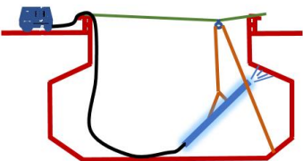
B.清洗舱顶部倾斜面，组装14米“长龙”，大倾角清洗。
