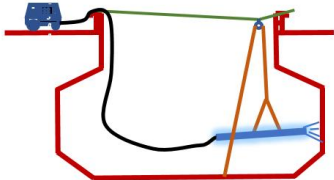
C.清洗舱下立面，组装8米“长龙”，基本保持垂直面清洗。
